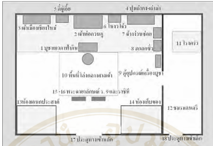
รูปที่ 3 แผนผังศาลเจ้ากวนอู
